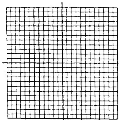
图 1 栅格图
